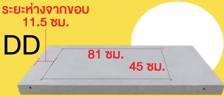
โดมอนด์ เคาน์เตอร์ ซิงค์หลุมคู่ Diamond Counter Double Sink *ขนาดเจาะช่องมาตรฐาน
